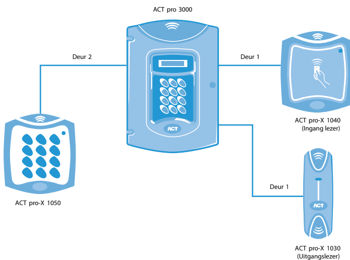
Schema voor ACT pro-X lezer
